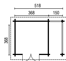
368×368 cm + 150 cm mit seitlich integriertem Unterstand, mit 45 mm BB
