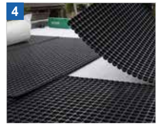
4 *Drän- und Speicherplatte 20 mm Platten ca. 1,06 x 2,36 m
