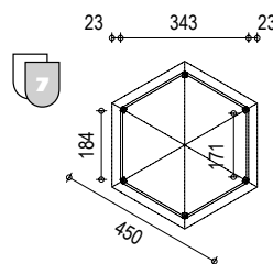
Modena Typ 2 6-Eck-Pavillon, offen
