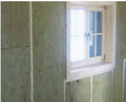
„Winterfest-Option“: doppelschalige Außenwand mit innenliegender Dämmung. Aufpreis für doppelschalige Außenwände: Verschiebesystem und ca. 18 mm Nut- und Federbretter inkl. Befestigungsmaterial und breiteren Tür- und Fensterfutterrahmen; geeignet für Einbringung von ca. 100 mm Dämmmaterial
