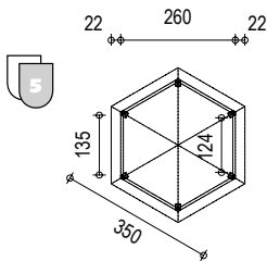
Modena Typ 1 6-Eck-Pavillon, offen
